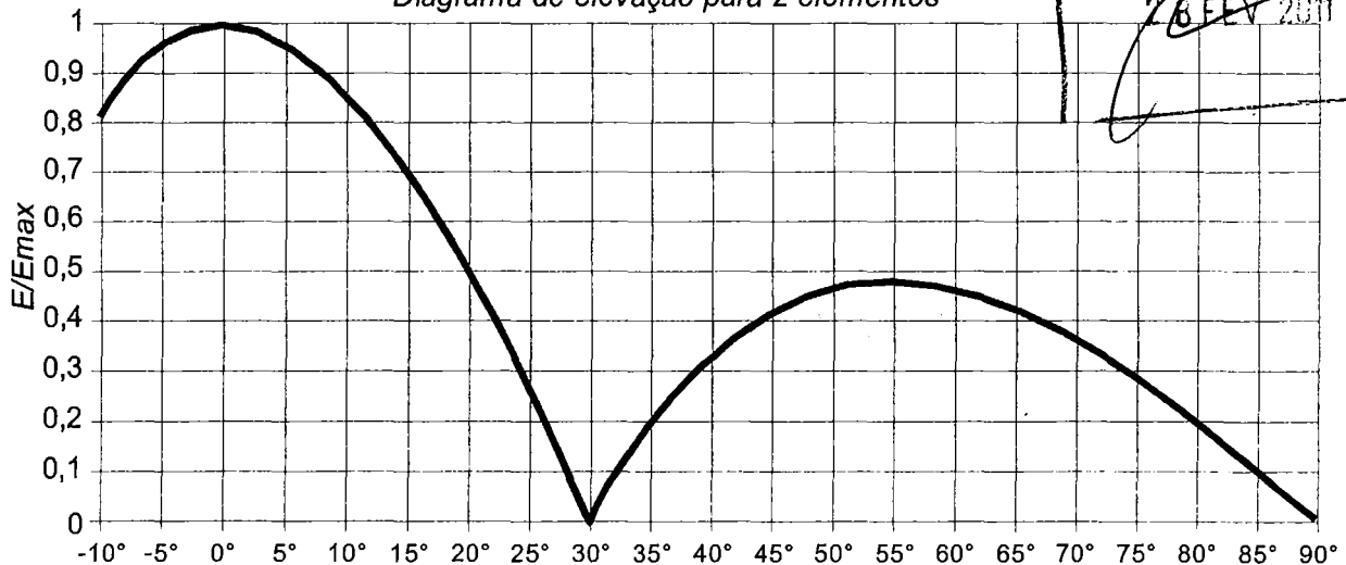
Antena para transmissão em FM modelo COLINEAR Diagrama de elevação para 2 elementos
