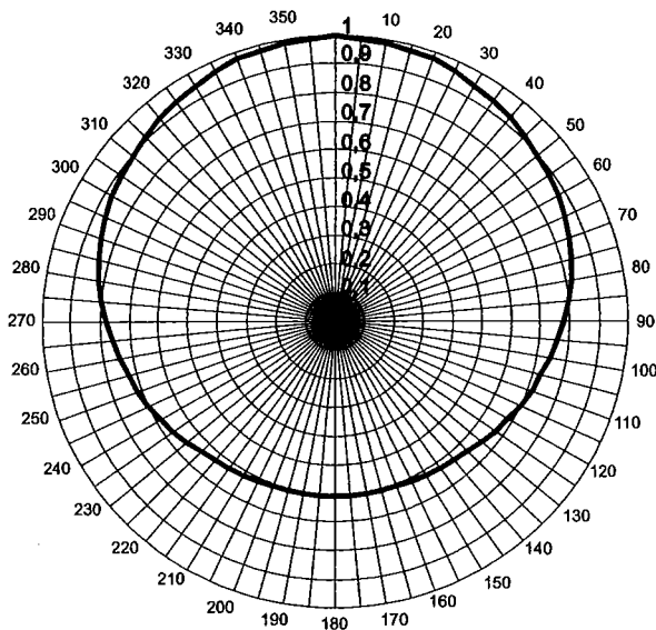
Diagrama de Elevação para 1 elemento
