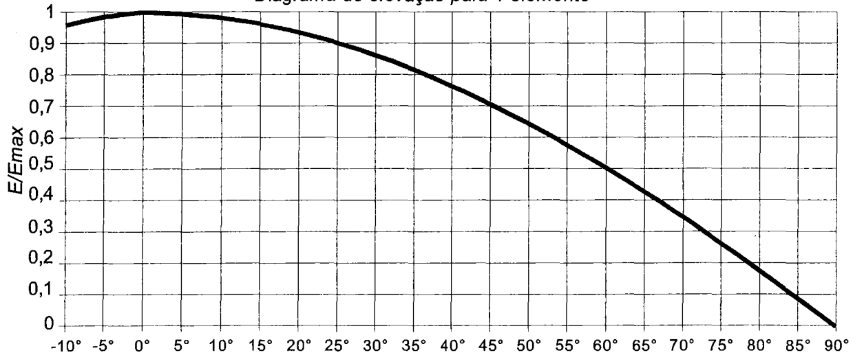
Antena para transmissão em FM modelo COLINEAR Diagrama de elevação para 1 elemento
