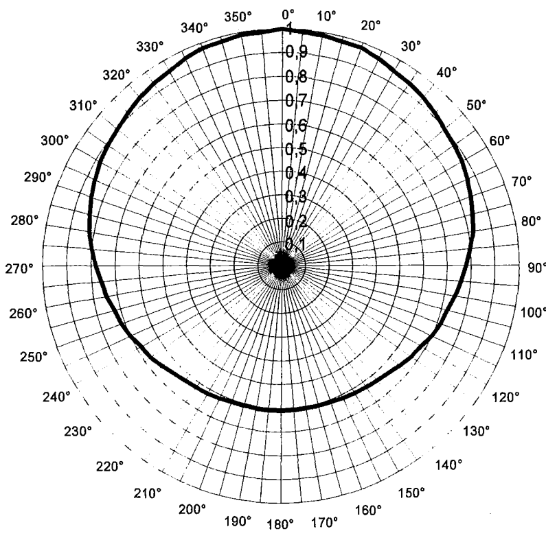
Antena Colinear para FM Diagrama na polarização vertical - Ângulo de 1/2 pot.: 220°
