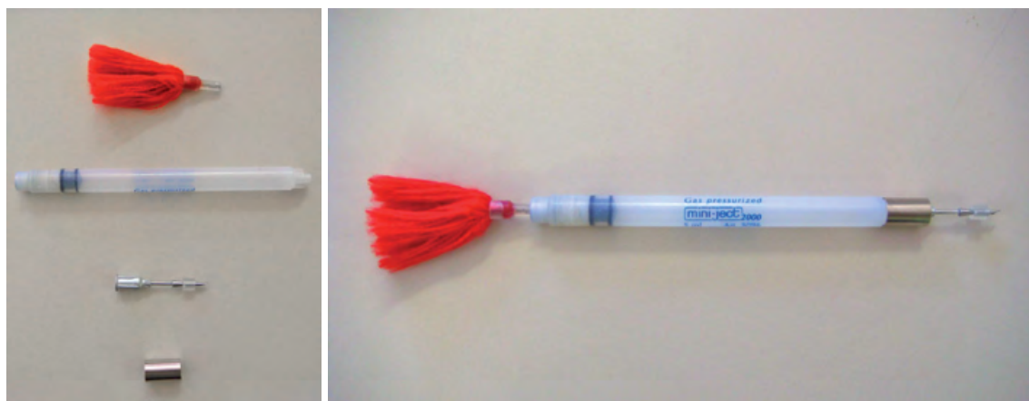
Figura 19 – Componentes do dardo e montagem
