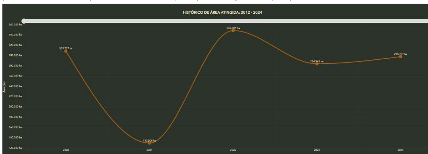
Figura 3. Área total atingida por fogo de manejo nas unidades de conservação fedearais nos anos de 2020 a 2024. Fonte: Vellozia/DGEO/CGPRO/ICMBio
