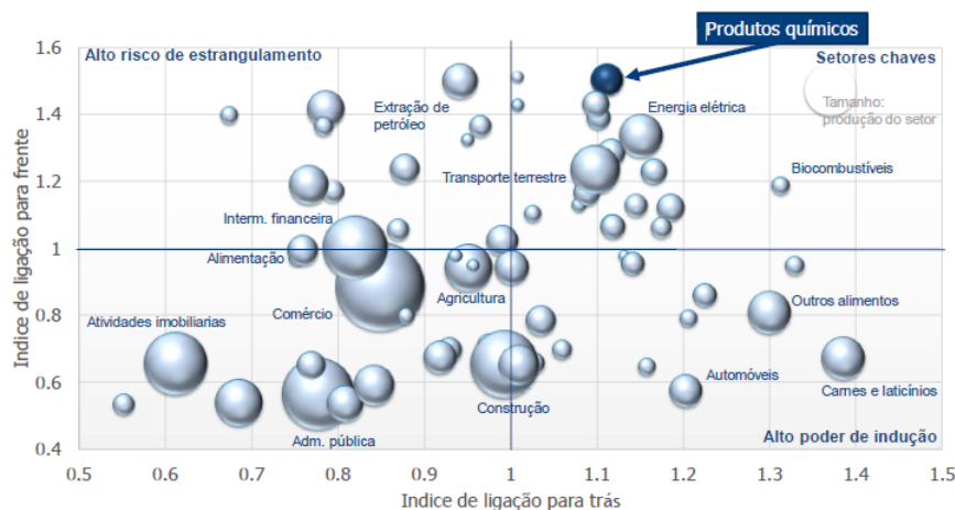
Gráfico 2.1: Interligações setoriais
