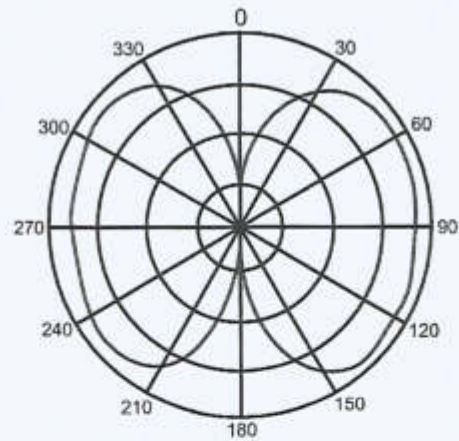
Diagrama de polarização vertical
