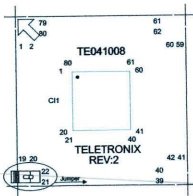
Figura5. Vista Superior Microcontrolador
