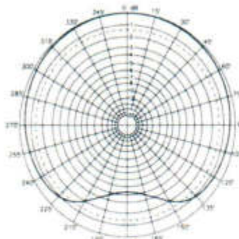
Diagrama de Irradiação Horizontal
