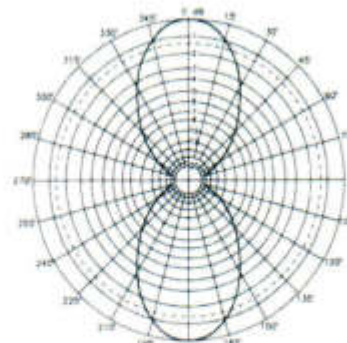
Diagrama de Irradiação Vertical
