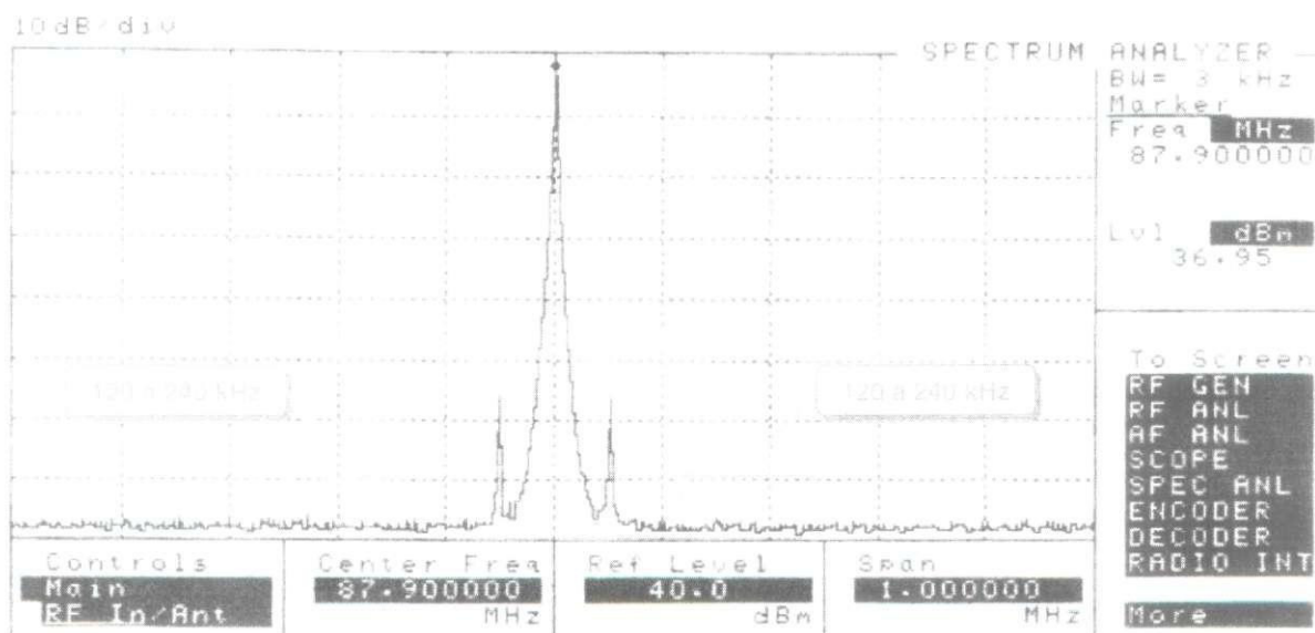
Figura 2 - Frequências afastadas de 120 a 240 kHz
