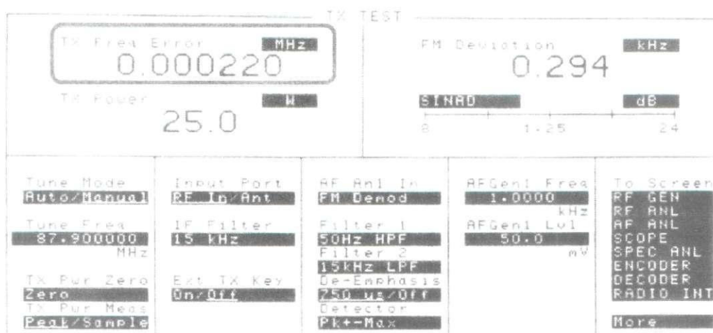
Figura 1 – Tolerância de frequência
