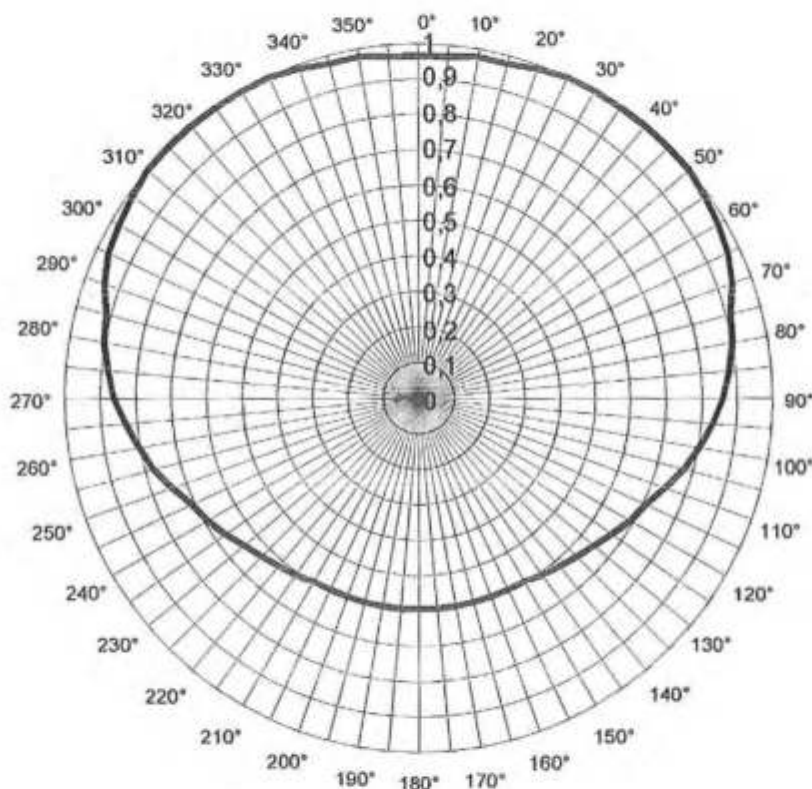
Antena Modelo FM CIRO Diagrama de irradiação horizontal na polarização vertical
