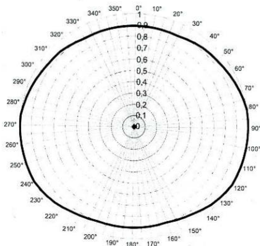
Antena Modelo FM Espiral Diagrama horizontal na polarização vertical
