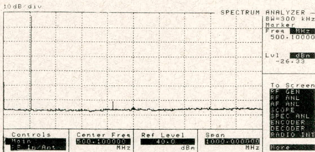
Figura 4 - Frequências afastadas de mais de 600 kHz
