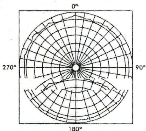
Diagrama de Irradiação (Horizontal)
