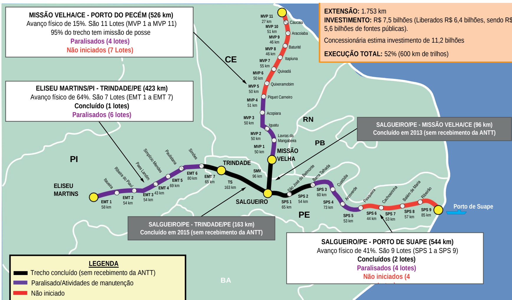
Figura 6 - Situação das obras da Transnordestina
