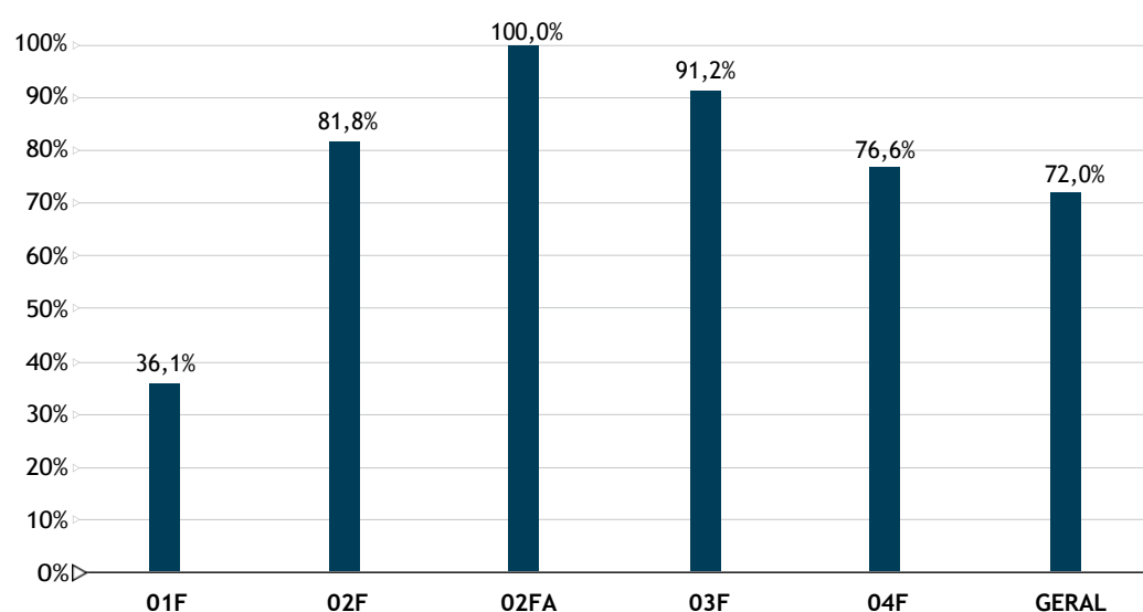
Gráfico 2 - Grau de avanço das obras do trecho Caetité-Ilhéus da Fiol (setembro 2017)
