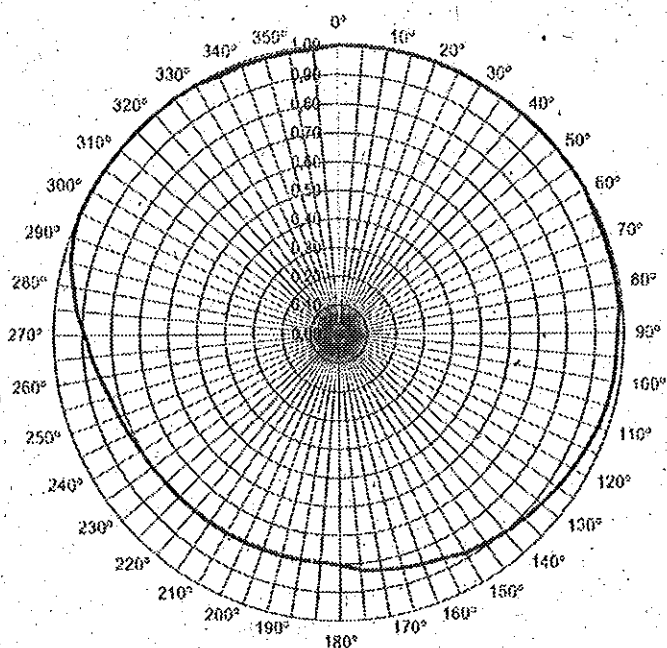
Diagrama de Azimute Polarização Vertical
