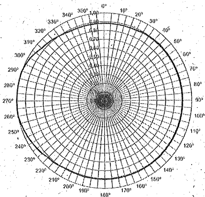
Diagrama de Azimute Polarização Horizontal
