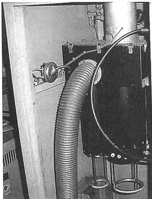
SAÍDA DE RF - EXCITADOR 100 W E CAVIDADE PARA 1 KW
