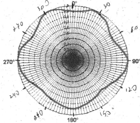
Padrão O - 360 de cobertura
