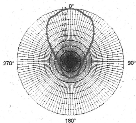
PADRÃO C - 80° de cobertura
