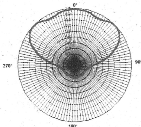
PADRÃO B - 140° de cobertura
