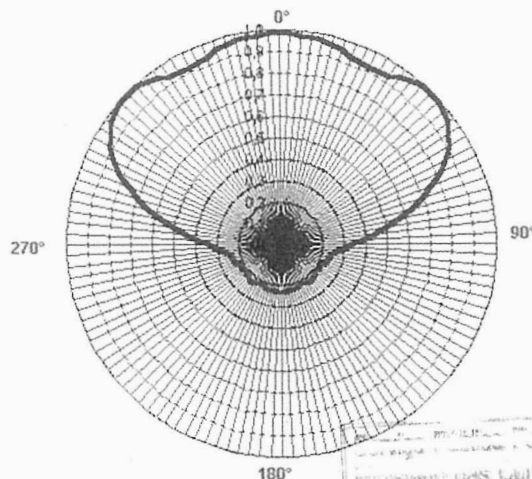
PADRÃO B - 140° de cobertura
