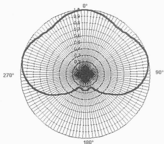
PADRÃO A - 220° de cobertura
