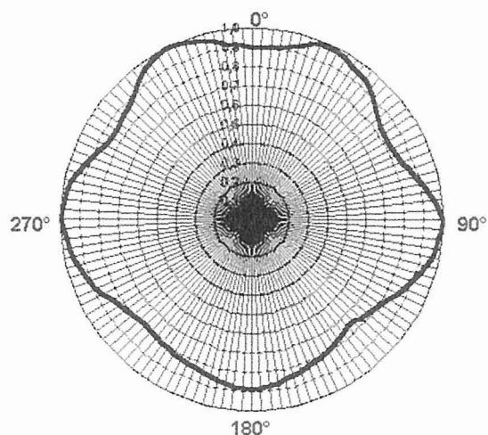
PADRÃO O - 360° de cobertura
