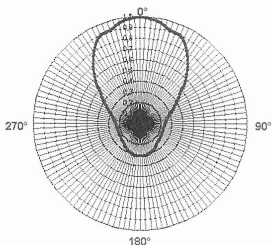
PADRÃO C - 80° de cobertura
