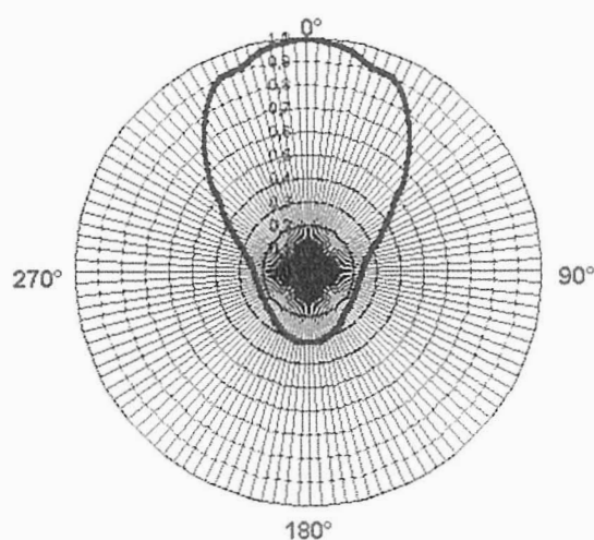
PADRÃO C - 80° de cobertura
