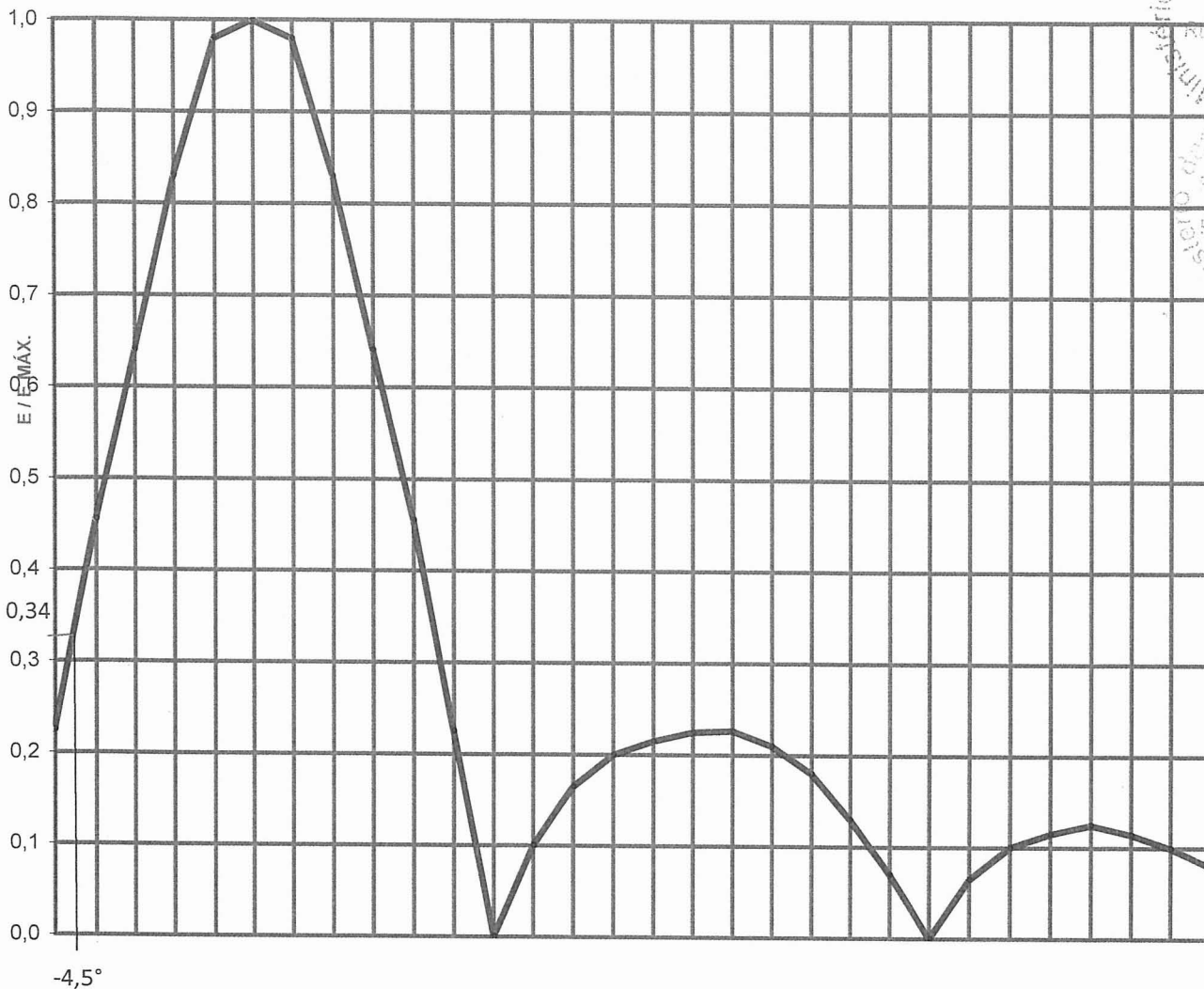
GRAUS - ABAIXO DA LINHA DO HORIZONTE
