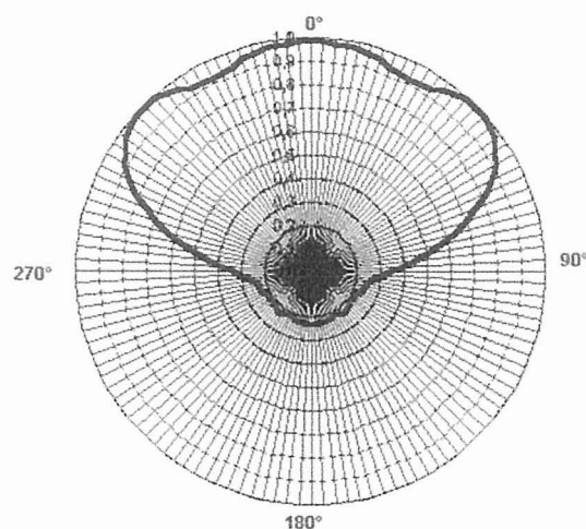
PADRÃO B - 140° de cobertura
