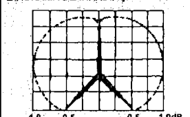
DIAGRAMA DE IRRADIAÇÃO VERTICAL
