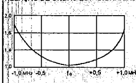
RELAÇÃO DE ONDAS ESTACIONÁRIAS
