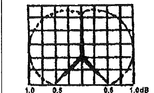
DIAGRAMA DE IRRADIAÇÃO VERTICAL
