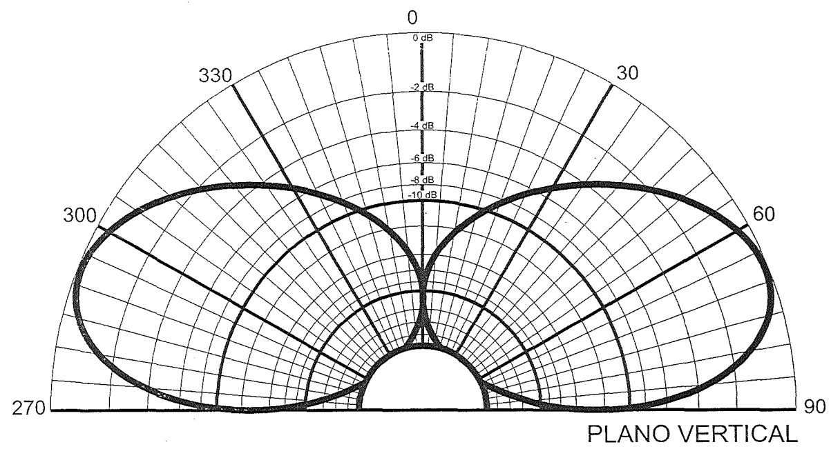
Ganho da Antena por Radial (Plano Vertical)
