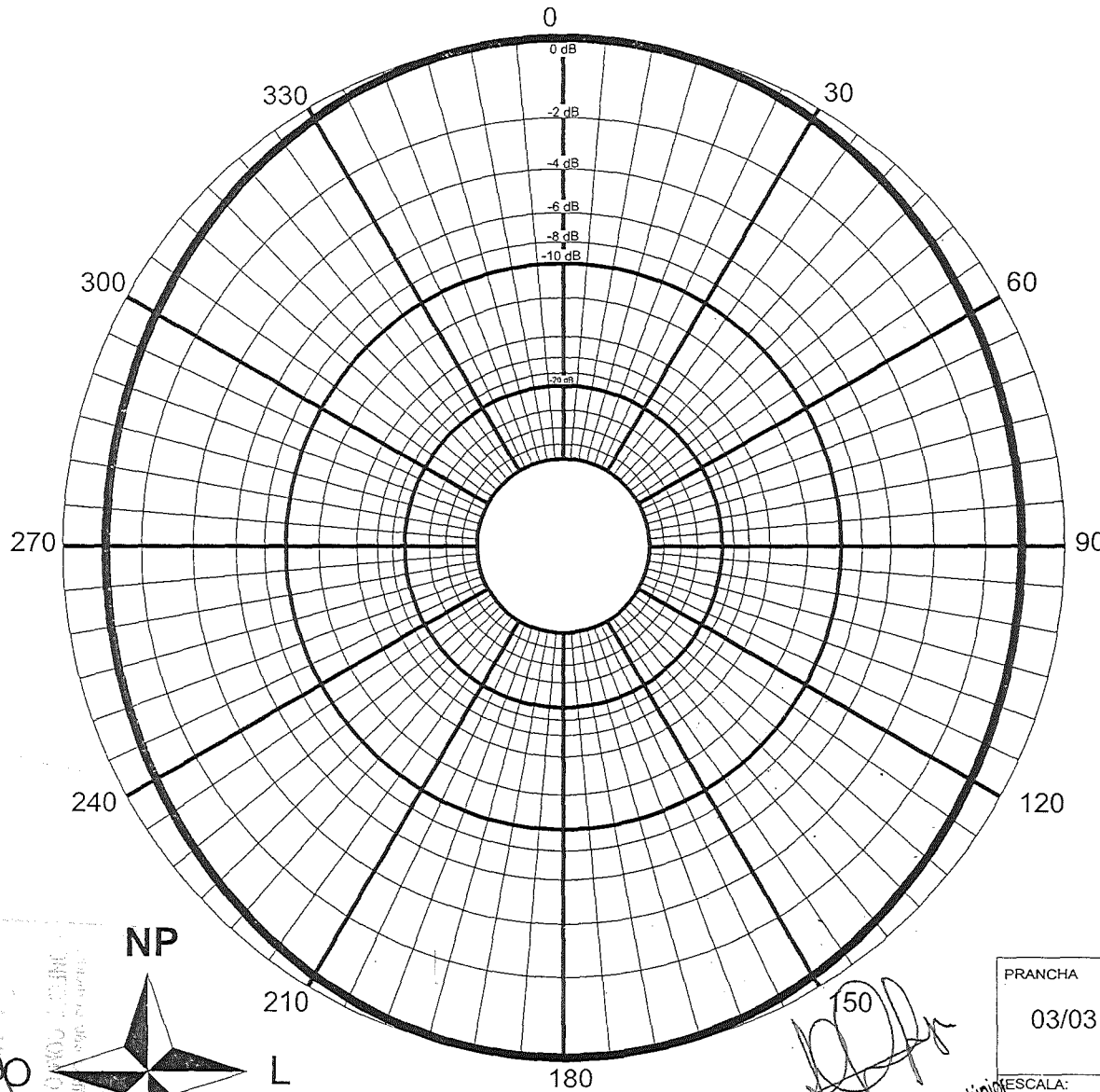
Ganho da Antena por Radial (Plano Horizontal)
