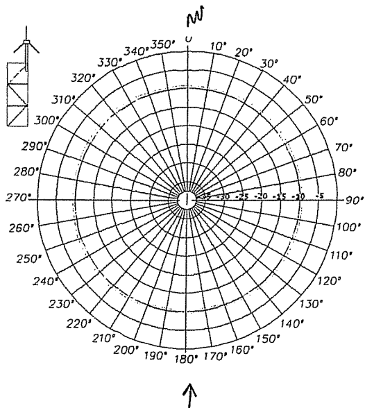
DIAGRAMA DE RADIAÇÃO HORIZONTAL Escala E/E max Montagem no Topo
