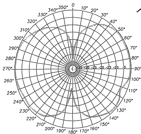
DIAGRAMA DE RADIAÇÃO VERTICAL Escala E/E max
