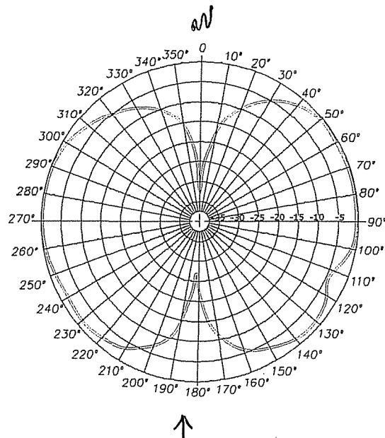
DIAGRAMA DE RADIAÇÃO VERTICAL Escala E/E max
