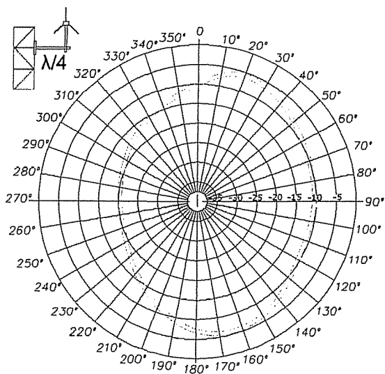
DIAGRAMA DE RADIAÇÃO HORIZONTAL Escala E/E max Montagem na Lateral a 1/4 Onda da Torre
