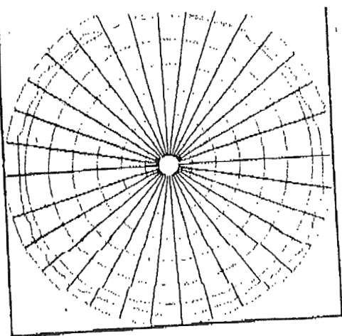
Diagrama de Irradiação (Horizontal)
