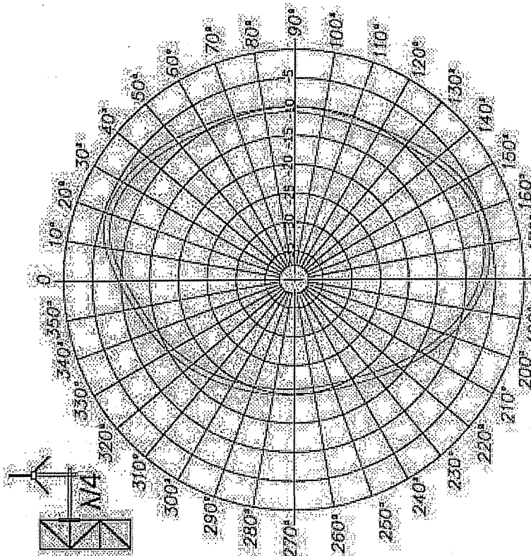
DIAGRAMA DE RADIAÇÃO HORIZONTAL Escala E/E max Montagem na Lateral a 1/4 Onda da Torre
