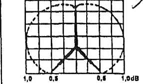
DIAGRAMA DE IRRADIAÇÃO HORIZONTAL
