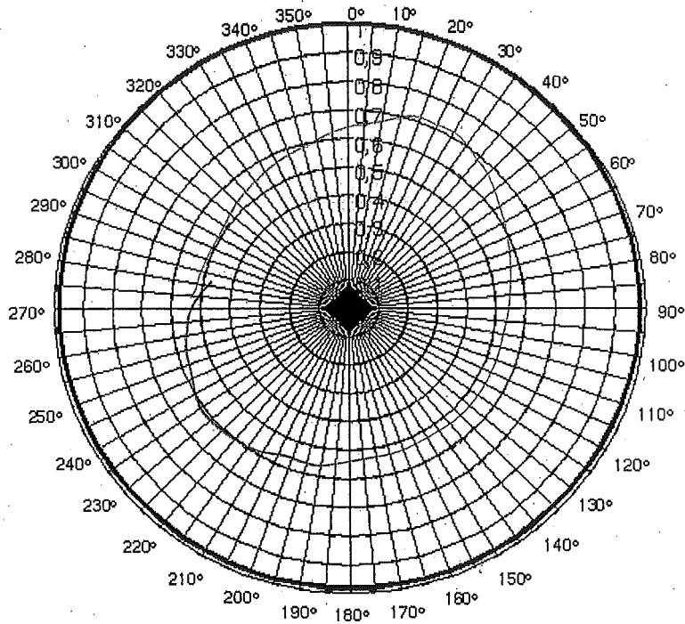
Antena para FM Plano Terra Diagrama de irradiação horizontal na polarização horizontal
