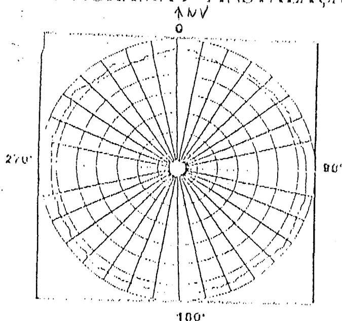
Diagrama de Irradiação (Horizontal)
