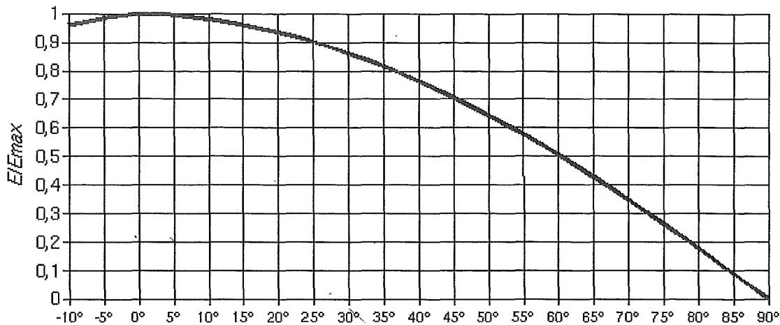
Antena para transmissão em FM modelo FMESPIRAL Diagrama de elevação para 1 elemento
