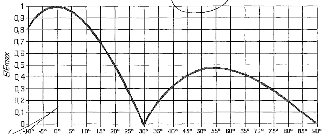
Antena para transmissão em FM modelo FMESPIRAL Diagrama de elevação para 2 elementos
