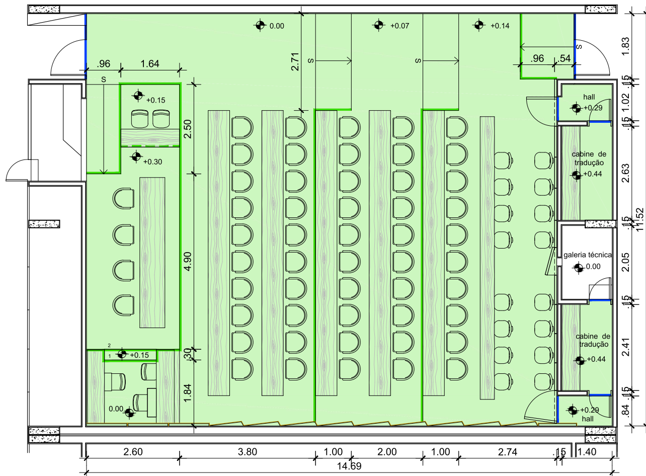
PLENÁRIO 3 PLANTA BAIXA esc 1/75
