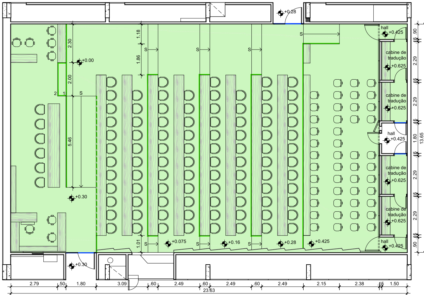
PLENÁRIO 1 PLANTA BAIXA esc 1/100
