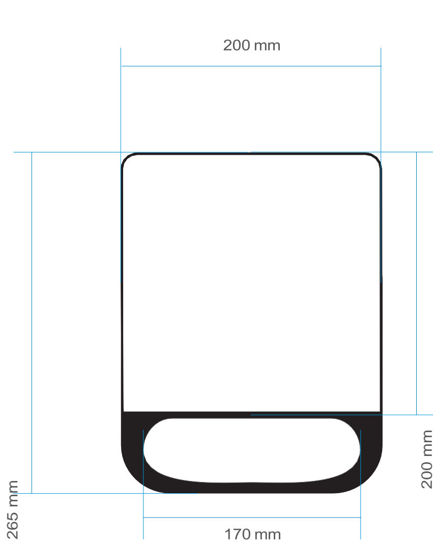
VISTA SUPERIOR
