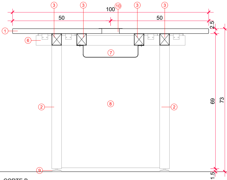
CORTE B
