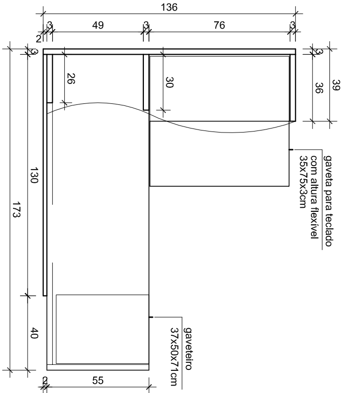
PLANTA BAIXA – h=78cm
