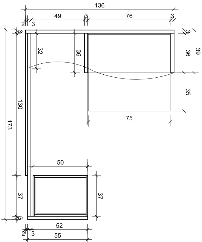
PLANTA BAIXA – h= 60cm
