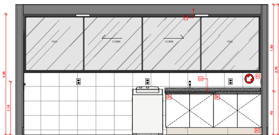
1 - A.S. - VISTA A-A 1:25
