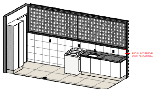
3 - A.S. - VISTA ISOMÉTRICA
