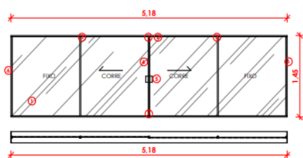
JANELA J6 | 517x120x130
