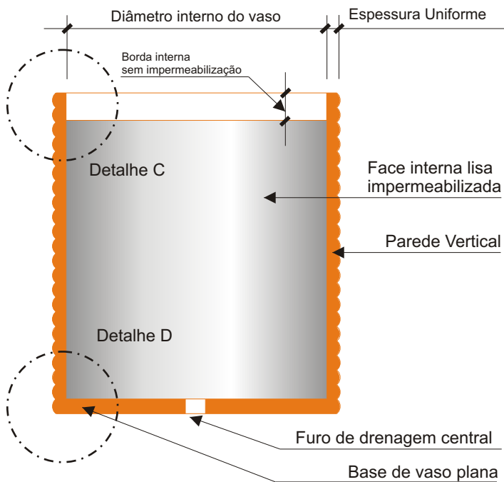
Seção Transversal
