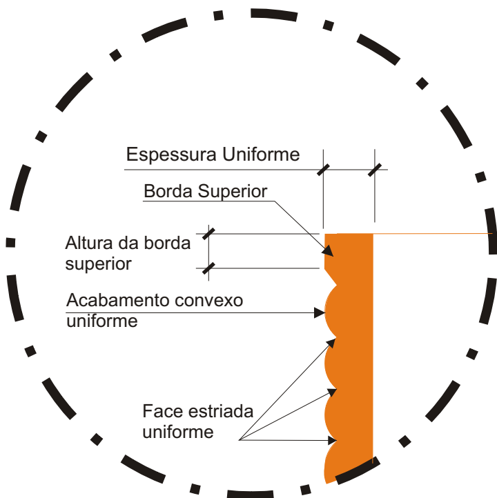
Detalhe A - Borda superior
