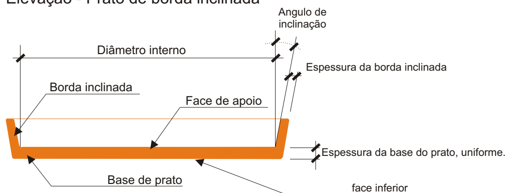
Elevação - Prato de borda inclinada
