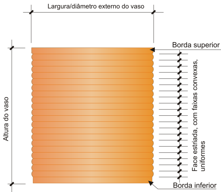
Vista Lateral
