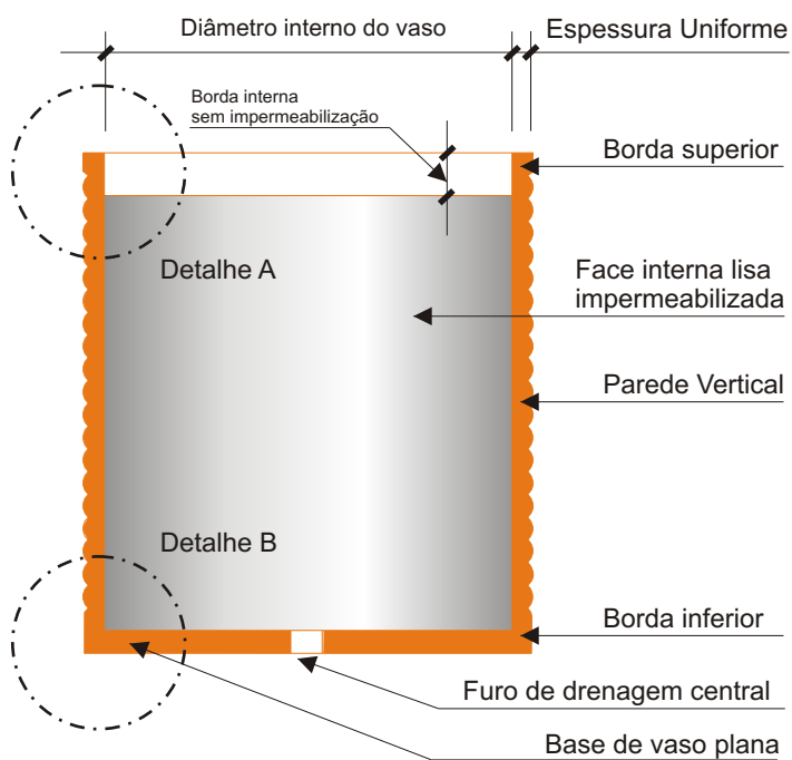
Seção Transversal
