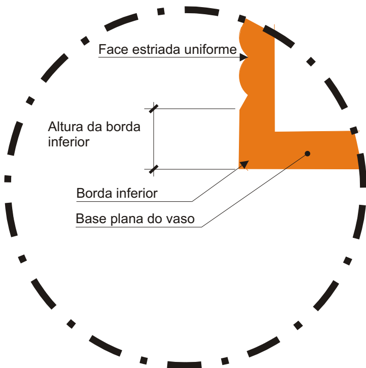
Detalhe B - Borda inferior
