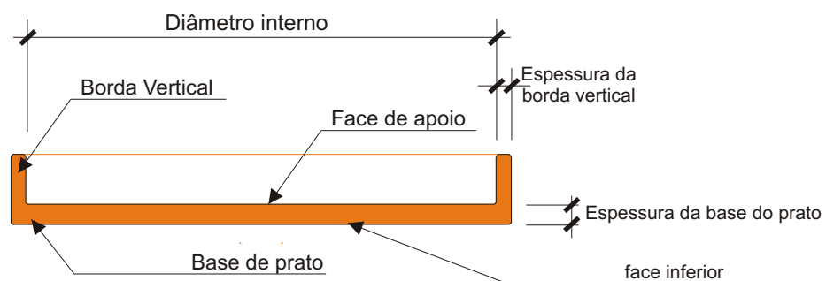
Seção - Prato circular de borda vertical
