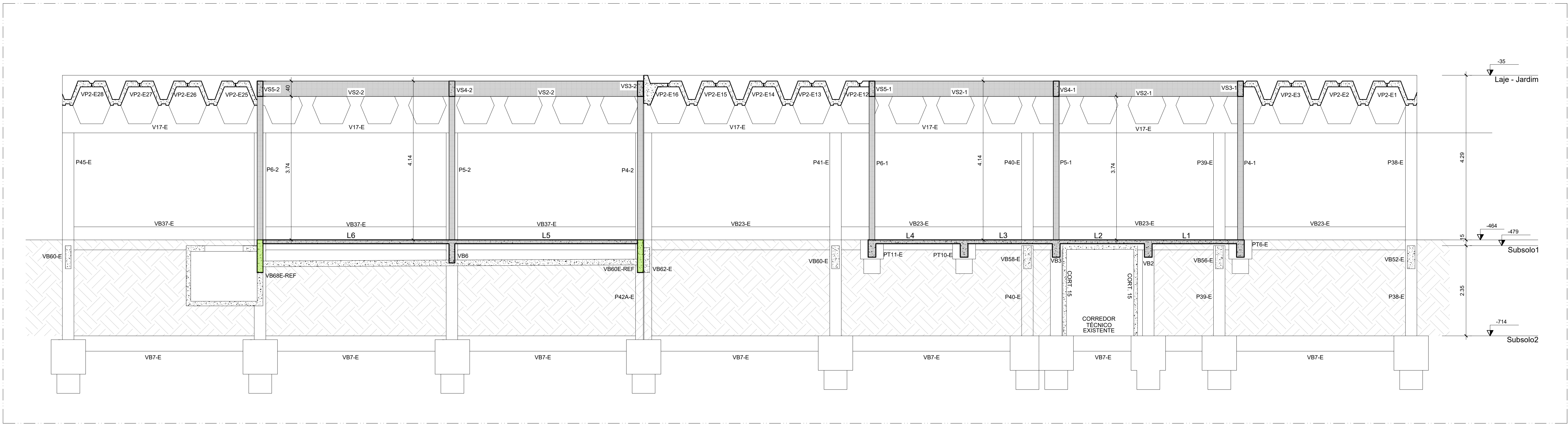
CORTE CC ESCALA 1:50
