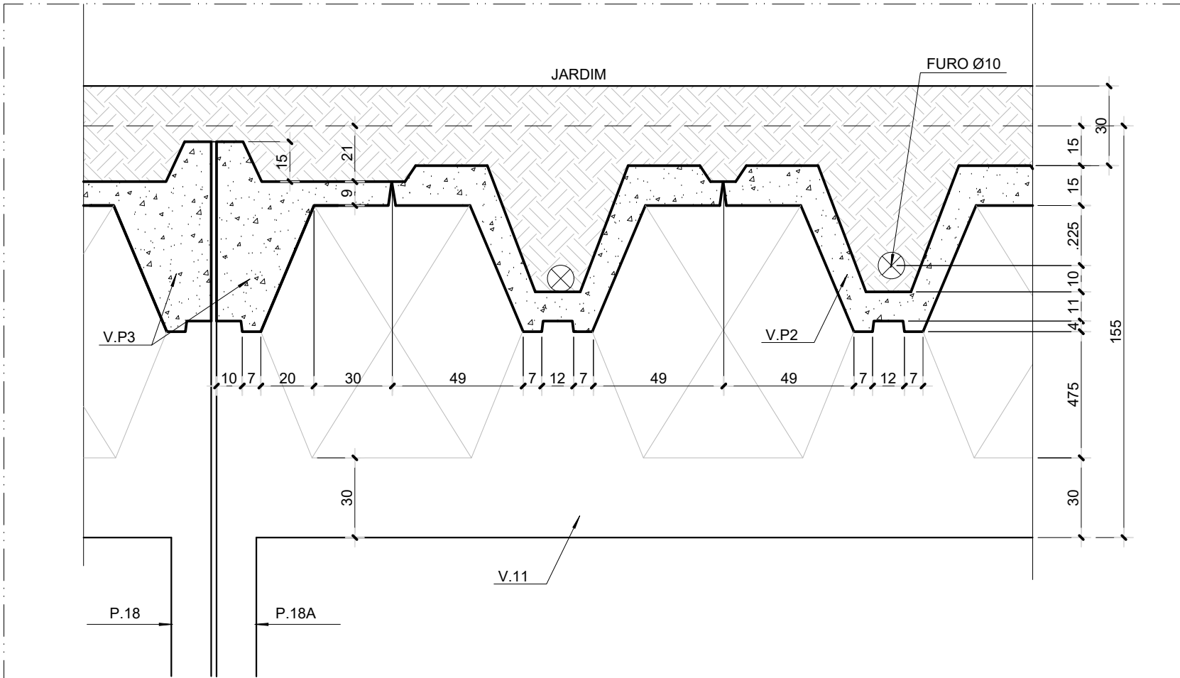
DETALHE DAS VIGAS V.11 E VP'S PAVIMENTO LAJE JARDIM -TÉRREO ESCALA 1:20
