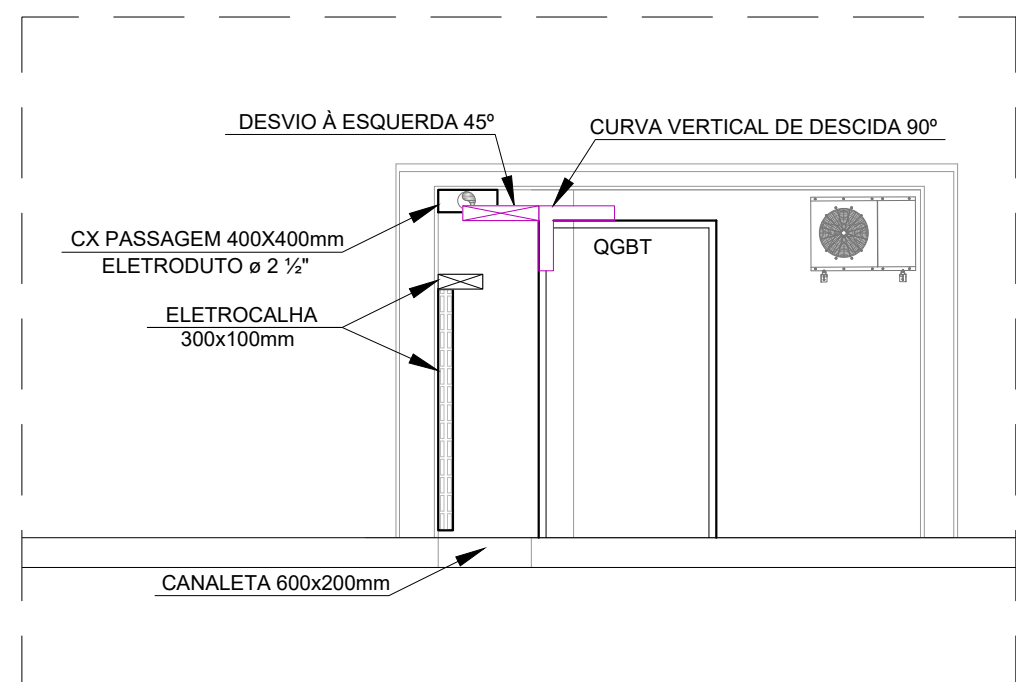
VISTA II - SALA QGBT, ESCALA 1:50
