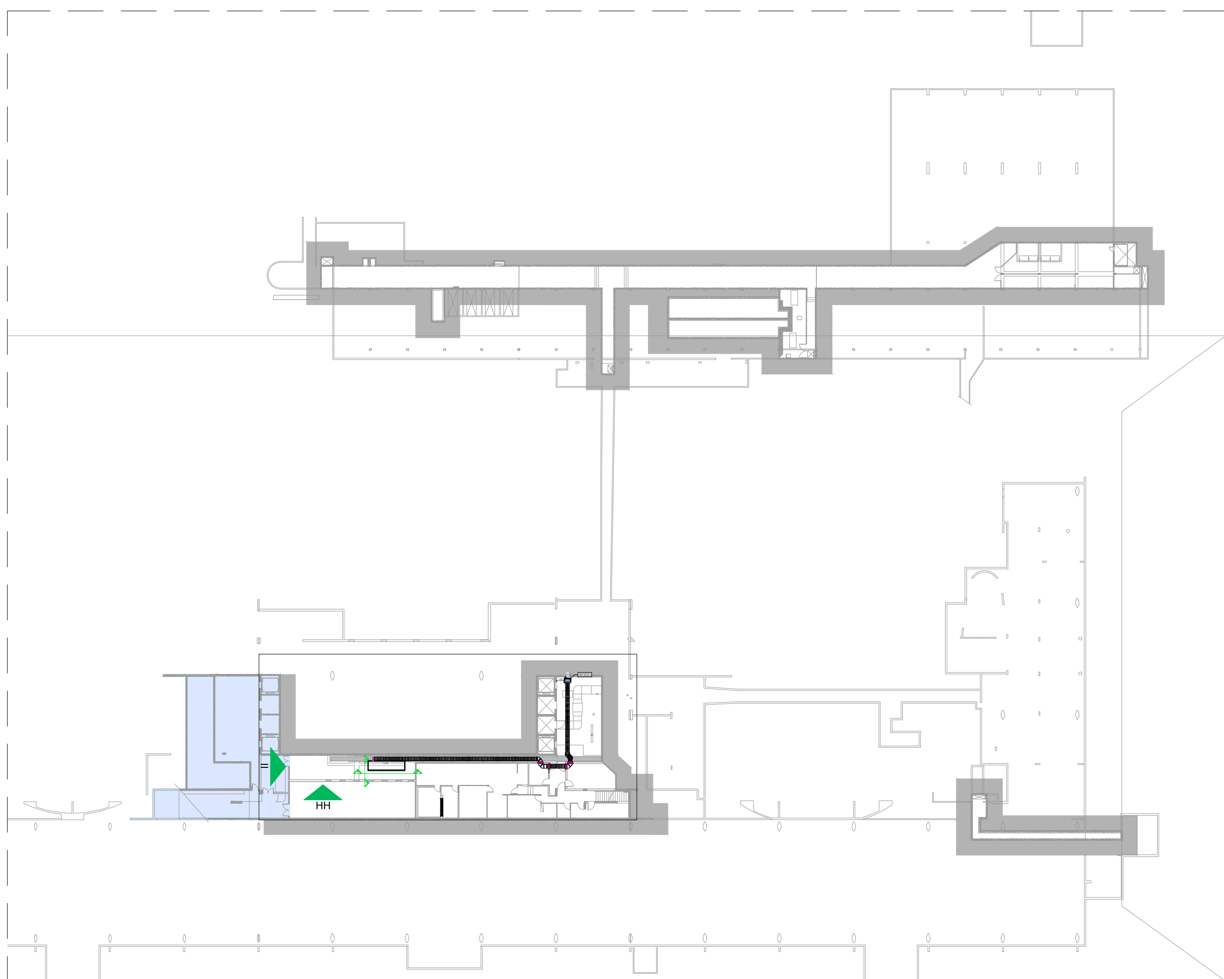
PLANTA BAIXA - 2º SUBSOLO - SALA DE QUADROS, ESCALA 1:500
