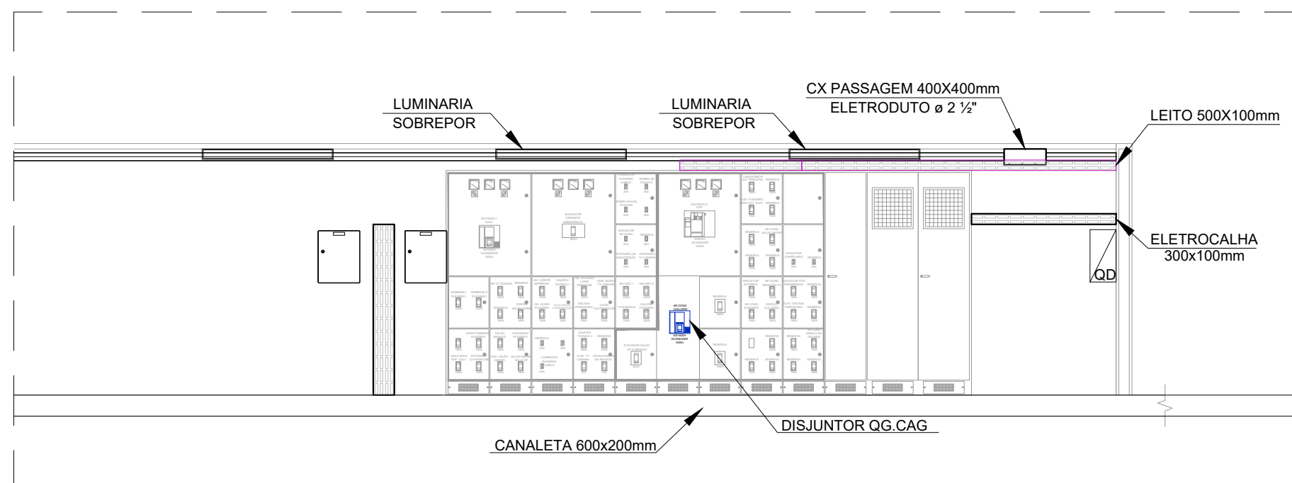
VISTA HH - SALA QGBT, ESCALA 1:50
