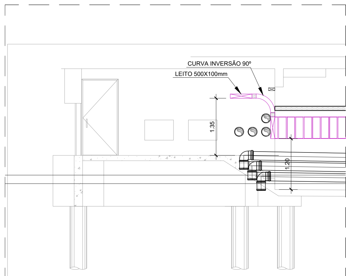
VISTA FF - SAÍDA CORREDOR GALERIA, ESCALA 1:50
