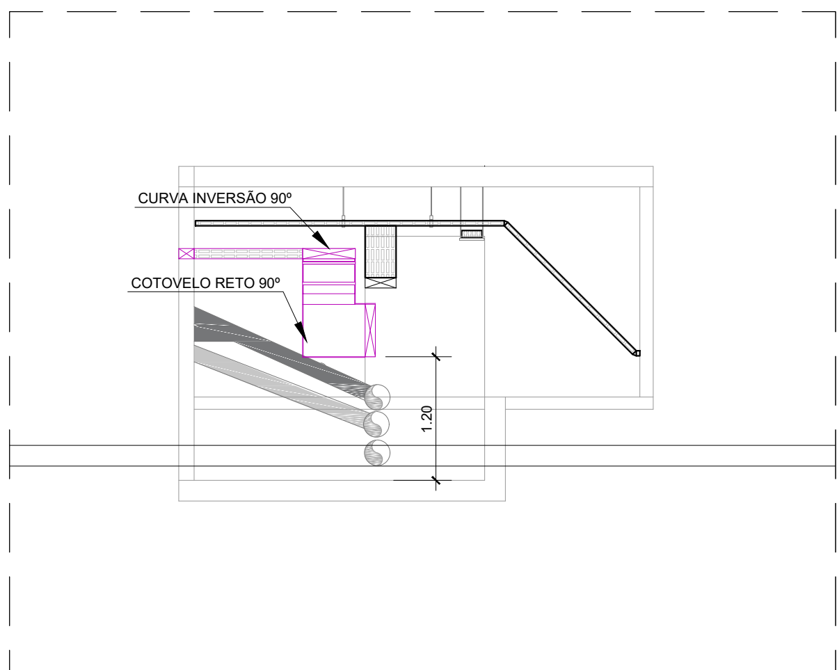
VISTA GG - SAÍDA CORREDOR GALERIA, ESCALA 1:50
