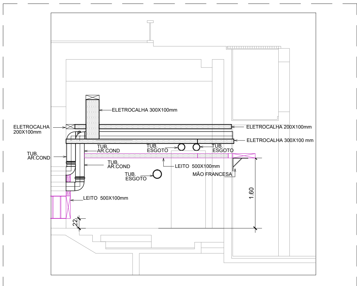
VISTA DD - ENTRADA CORREDOR GALERIA, ESCALA 1:50
