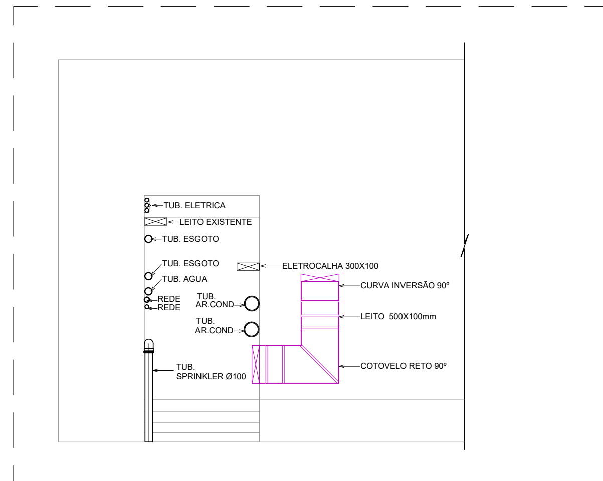
VISTA CC - SALA ENTRADA CORREDOR GALERIA, ESCALA 1:50
