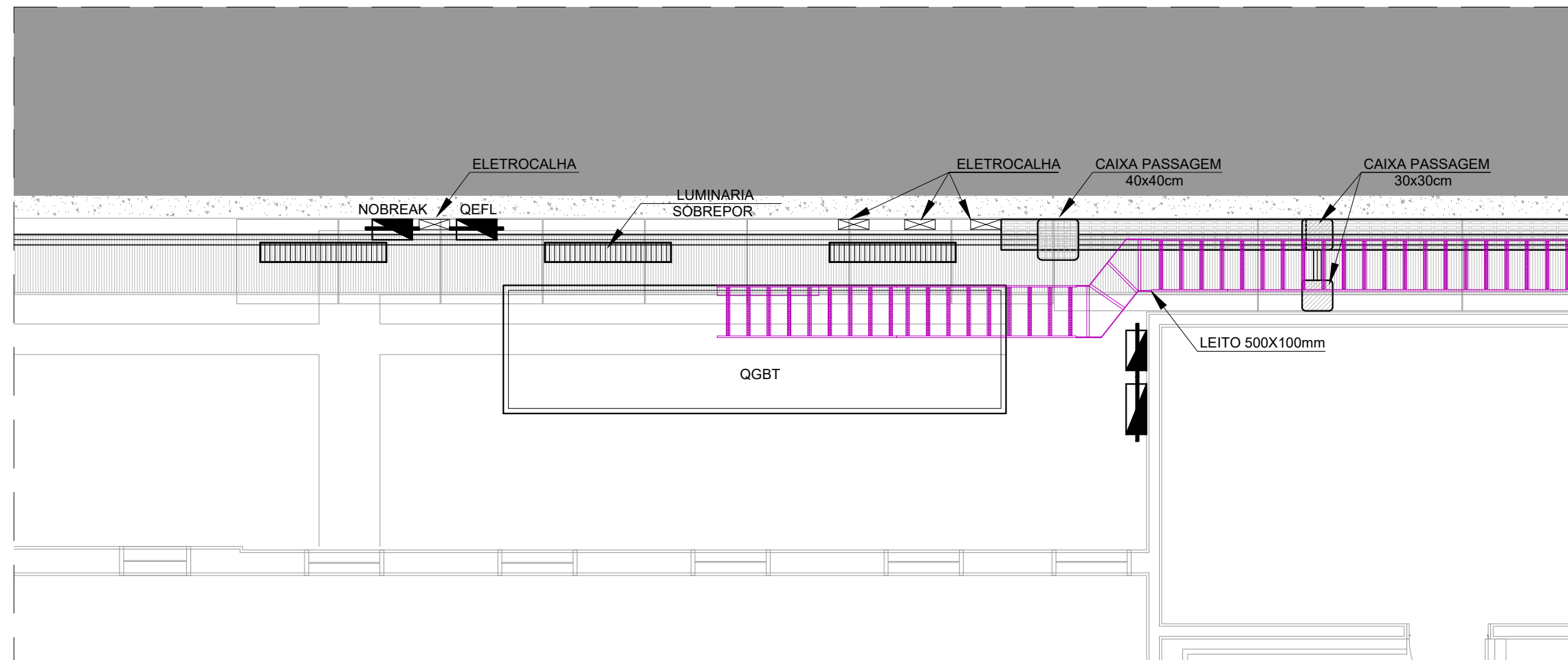
PLANTA BAIXA - SALA QGBT, ESCALA 1:50
