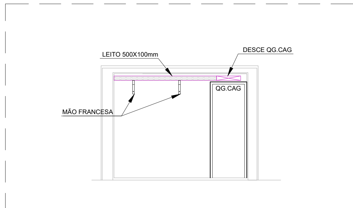
VISTA AA - SALA QG CAG, ESCALA 1:50
