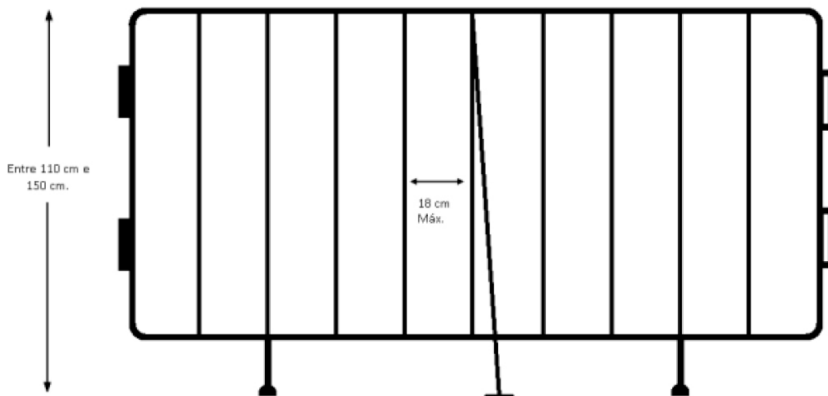
VISÃO FRONTAL
