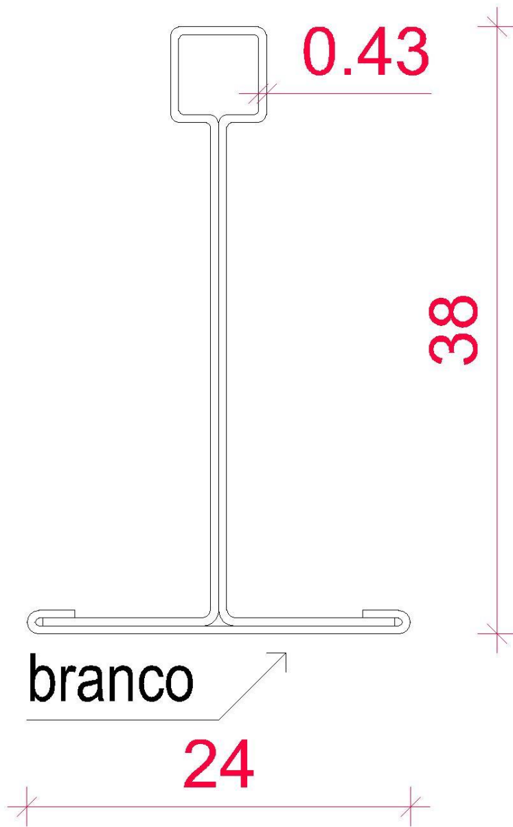
PERFIL T-24 medidas em mm
