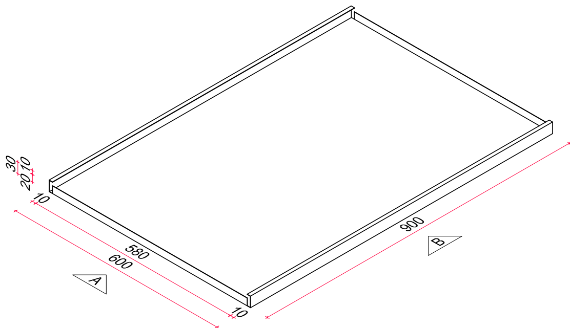
ISOMÉTRICO
