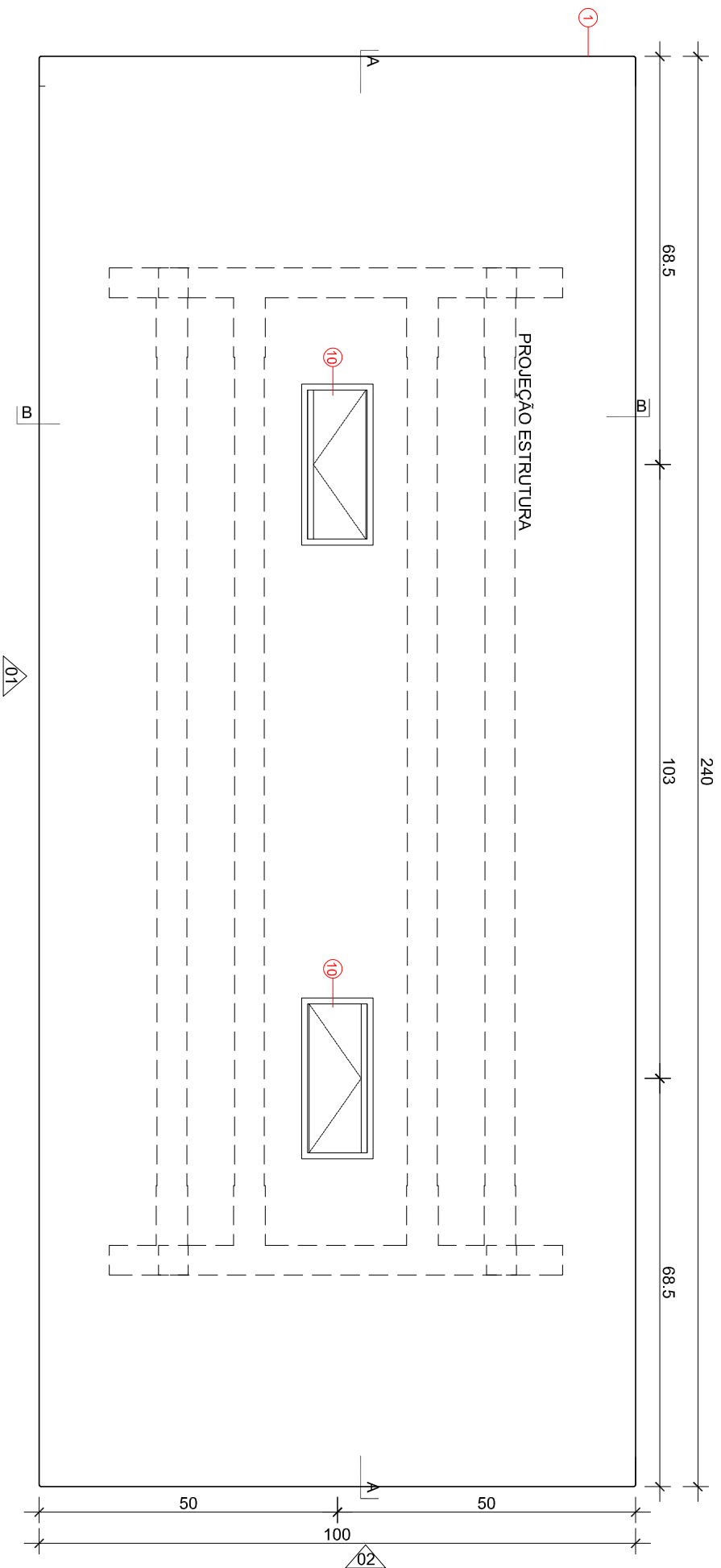
VISTA SUPERIOR
