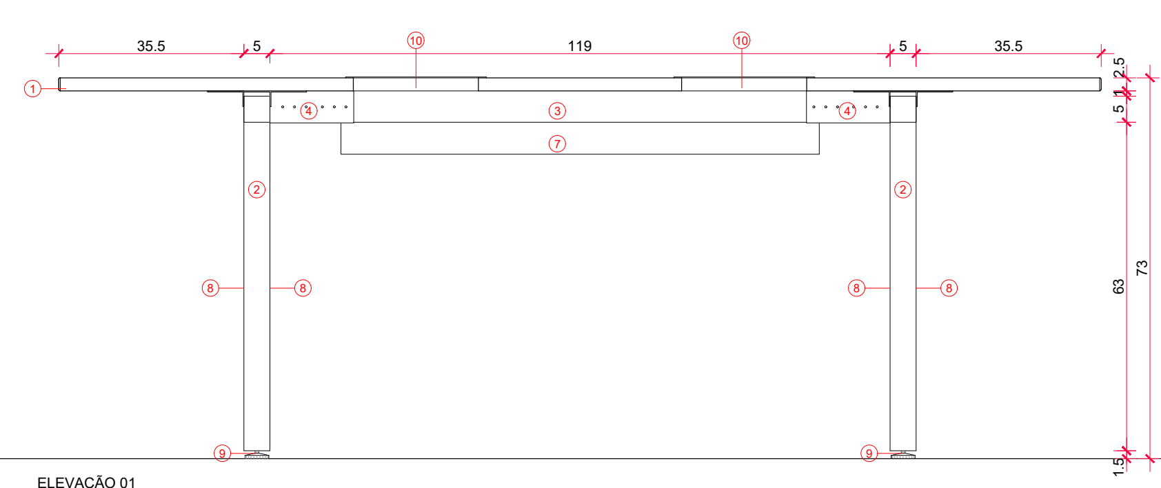
ELEVAÇÃO 01
