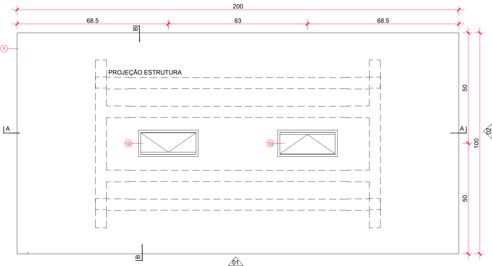
VISTA SUPERIOR
