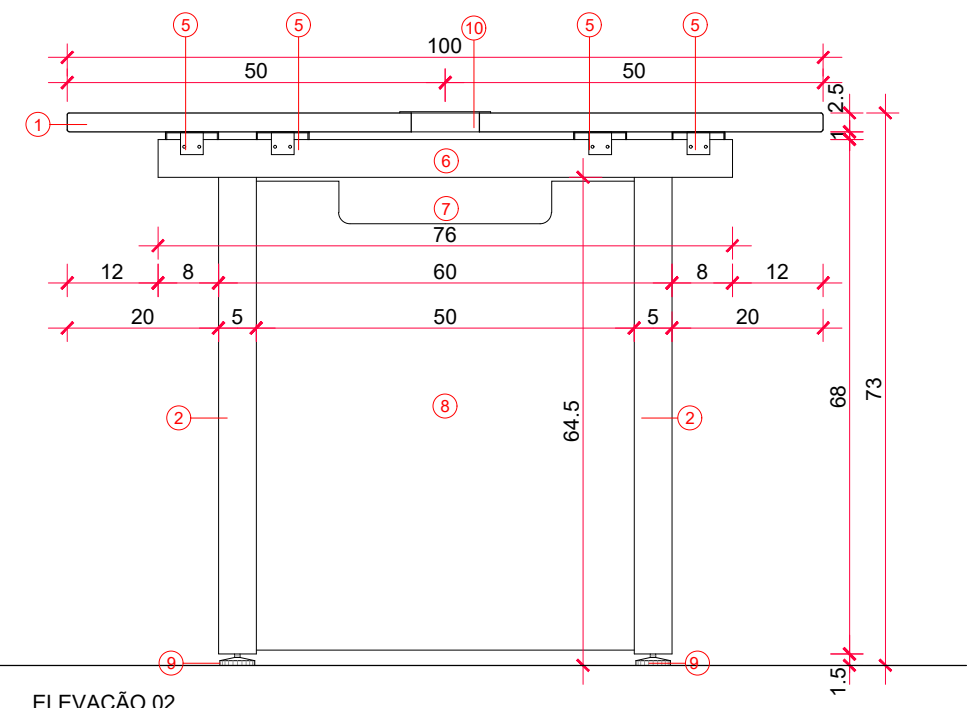
ELEVAÇÃO 02
