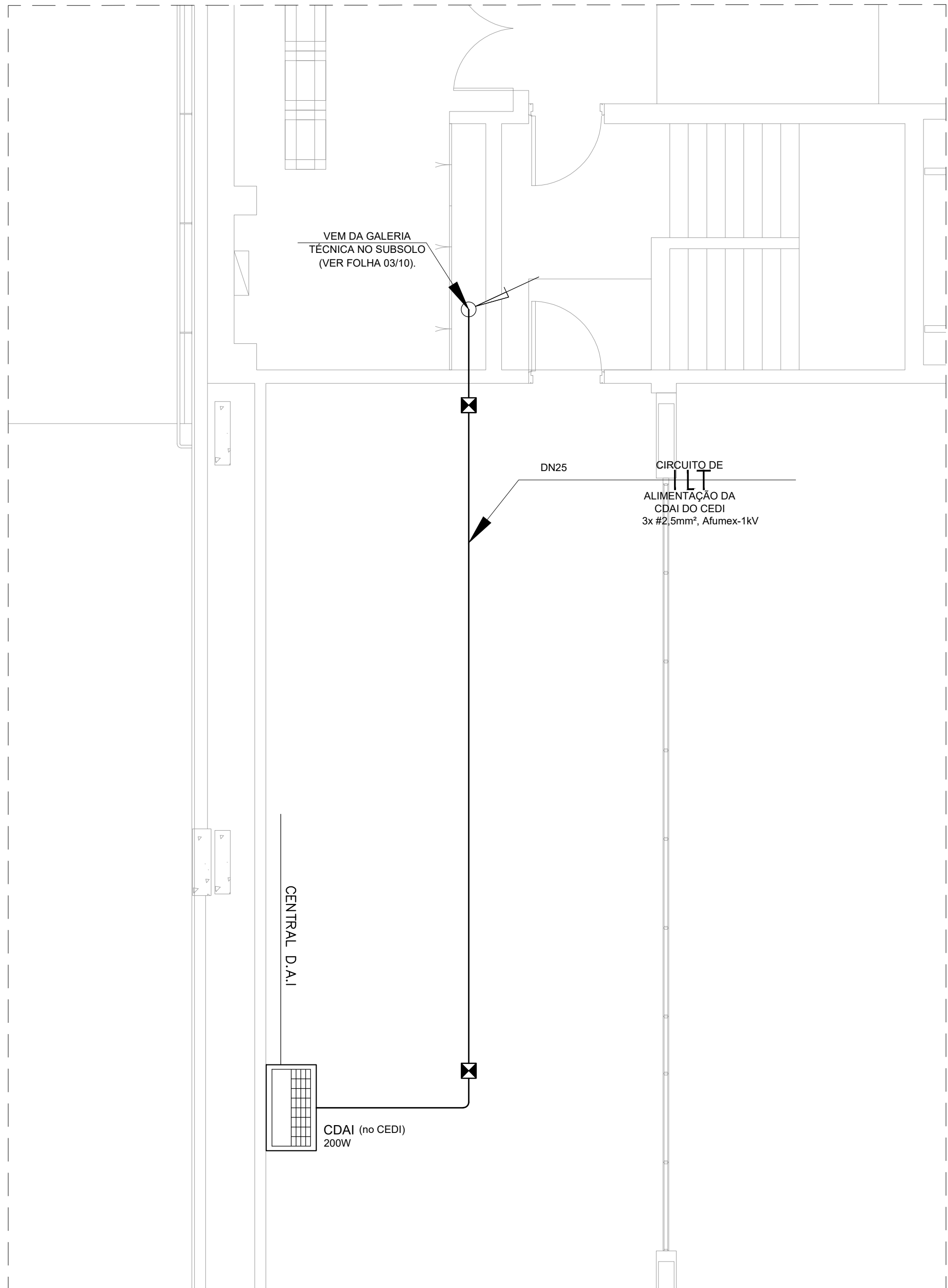
PLANTA BAIXA - ANEXO II 1º PAVIMENTO - ZOOM DA REGIÃO "C" ESCALA 1:50
