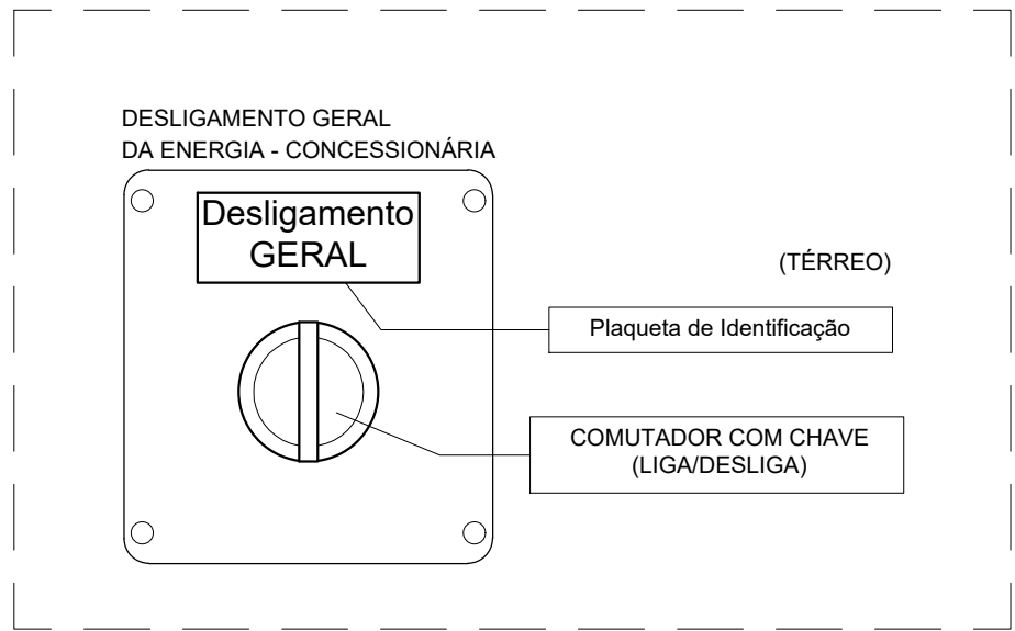
DETALHE SUGESTIVO DAS CAIXAS DE BOTOEIRAS DE COMANDO COM CHAVE DE DESLIGAMENTO DA ENERGIA - PARA ACIONAMENTO EM CASO DE INCÊNDIO PELO CBMDF SEM ESCALA
