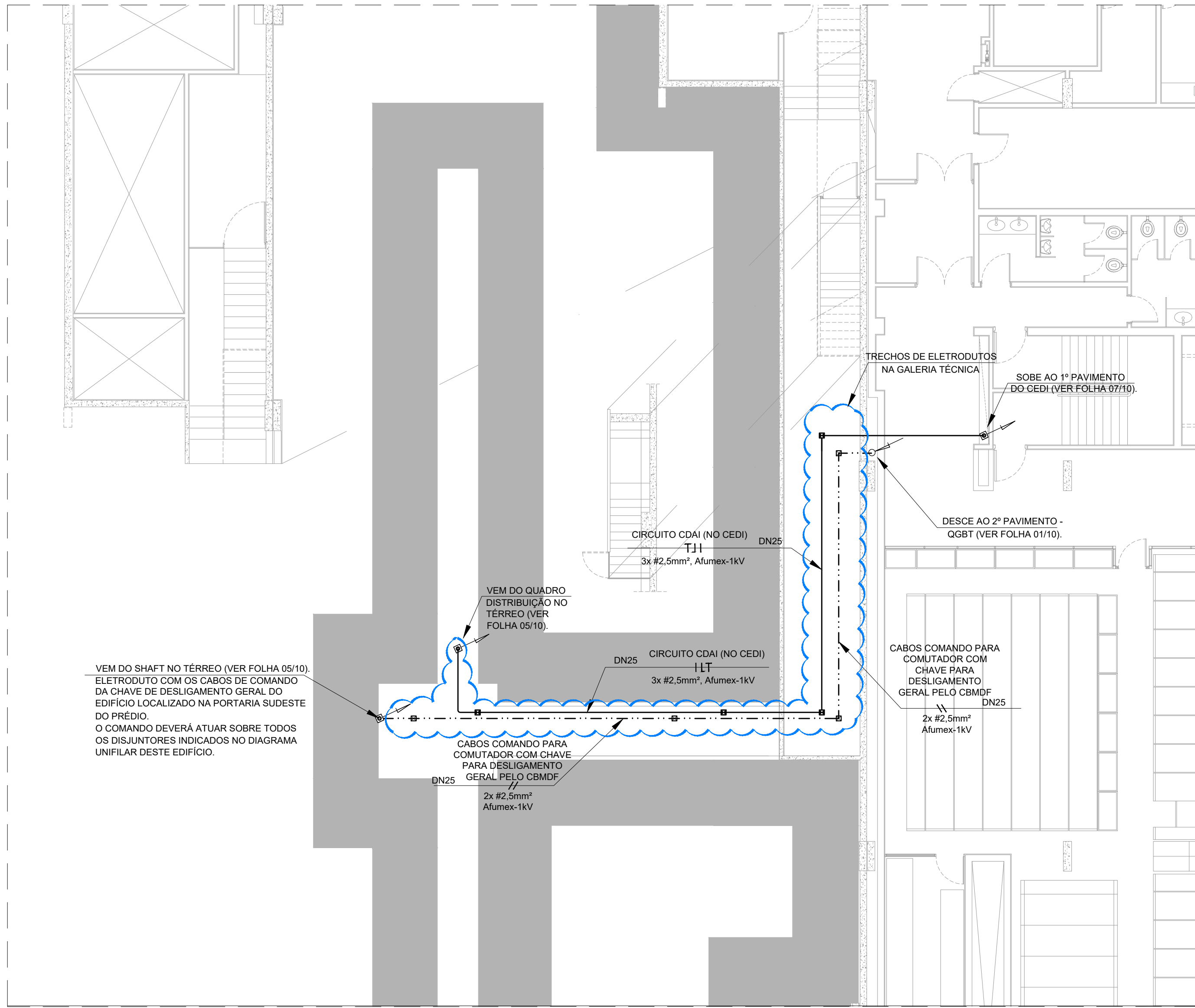
PLANTA BAIXA - ANEXO II - 1º SUBSOLO - (PARTE DAS REGIÕES "B,C") ESCALA 1:100
