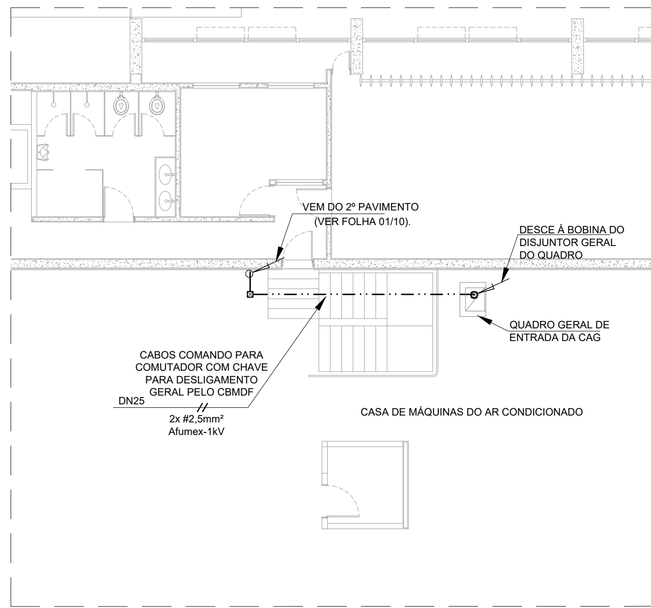
PLANTA BAIXA - ANEXO II - 1º SUBSOLO - (PARTE DA REGIÃO "C") ESCALA 1:100
